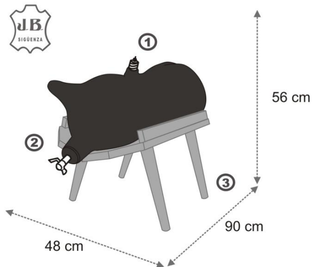
Figura 1. Especificaciones técnicas.
